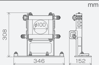
外形寸法 四面コアアタッチメント単体
