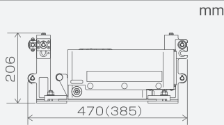
外形寸法 パワーボール取付状態 (両側)
