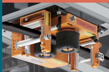
逆さ使いのケーブル落下防止
