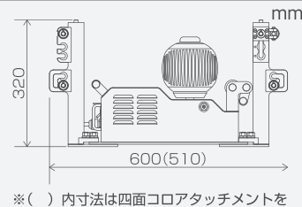
外形寸法 パワーボール取付状態 (両側)
