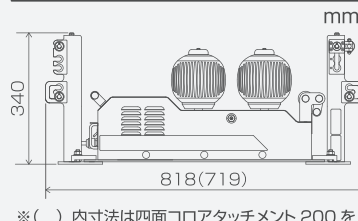
外形寸法 パワーボール取付状態 (両側)
