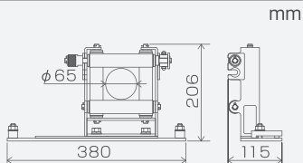
外形寸法 四面コアアタッチメント単体
