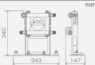
外形寸法 四面コアアタッチメント単体
